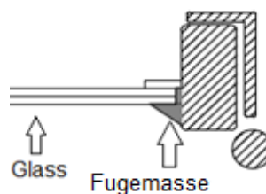
Snitt ved hengsler
