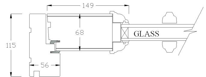
Element ytterdør med glass og Elite karm og sprosseprofil S2
