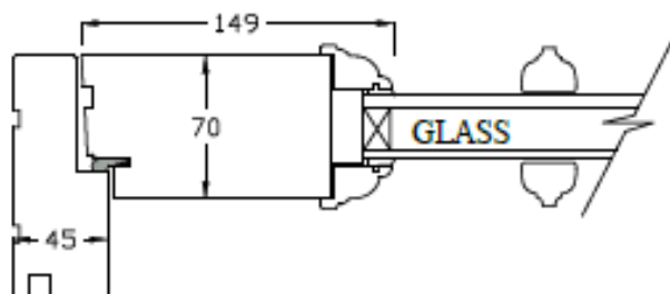
Element ytterdør med glass med griplistprofil P01 sprosseprofil S01 begge sider
