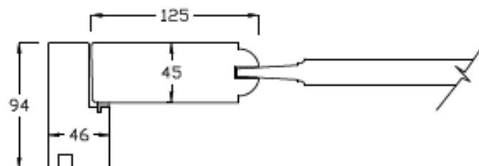
Ramtre innvendige dører Std innv ramtre profil Std friset fylling Std karm m/dempelist
