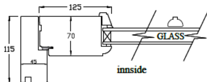
Ramtre ytterdør med glass Std P04 glasslister utv. Utenpåliggende S09 sprosser
