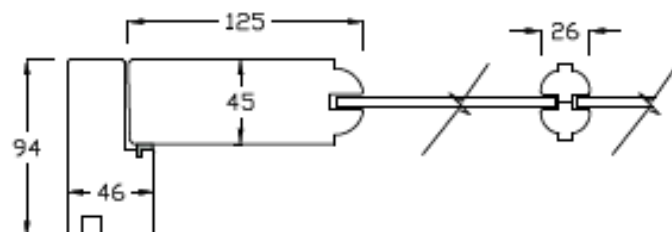
Ramtre innv.dører med glass ekte gjennomgående sprosser sprosseprofil S09
