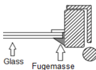
Snitt ved hengsler
