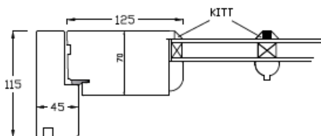
Ramtre ytterdør med ISOKITT glass Innv. sprosseprofil S09
